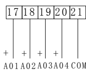
P/Q/I模拟量输出 P/Q/I Analog output
